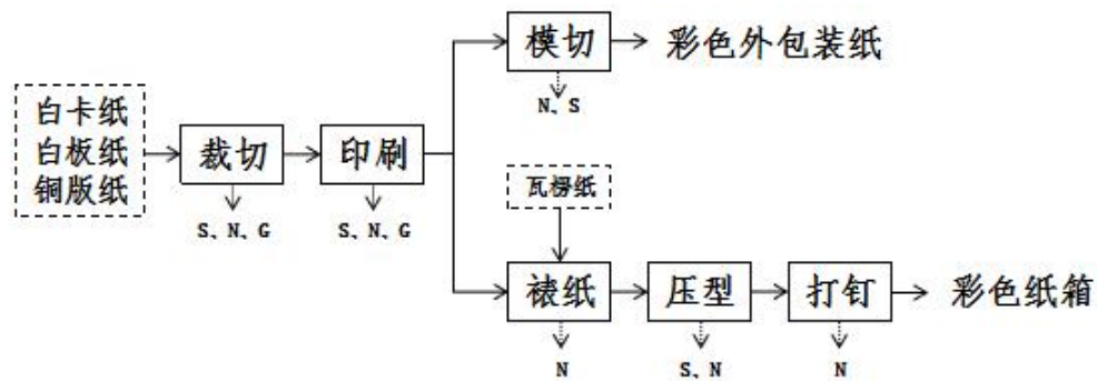
图 3-1 项目工艺流程及产污节点示意图
